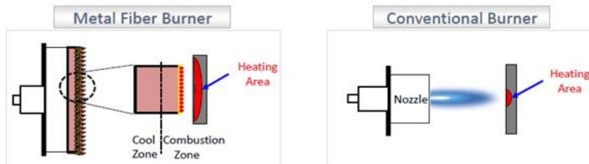
Şekil 2.28 : Gas brülör ve Infrared teknoloji ile ön ısıtma prosesi.
