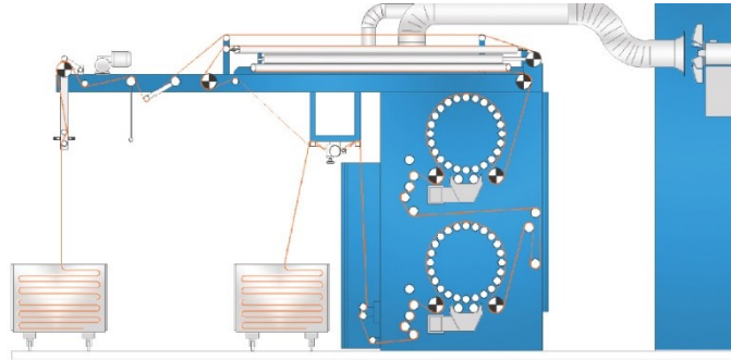
Şekil 2.11 : Şardon makinesi.
