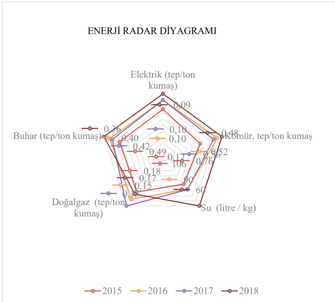
Şekil 3.6 : 2015-2018 yılları arası enerji radar diyagramı.
