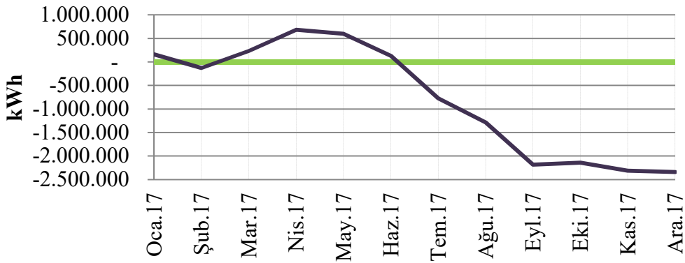
Şekil 3.4 : 2017 CUSUM grafiği.
